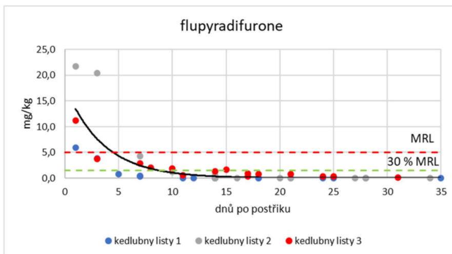
Obrázek 15 – Rychlost degradace úč. l. flupyradifurone v listech kedlubny.
